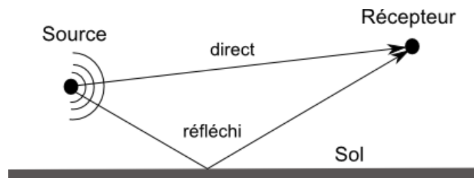
Figure 42 : influence du sol sur la propagation des ondes sonores
