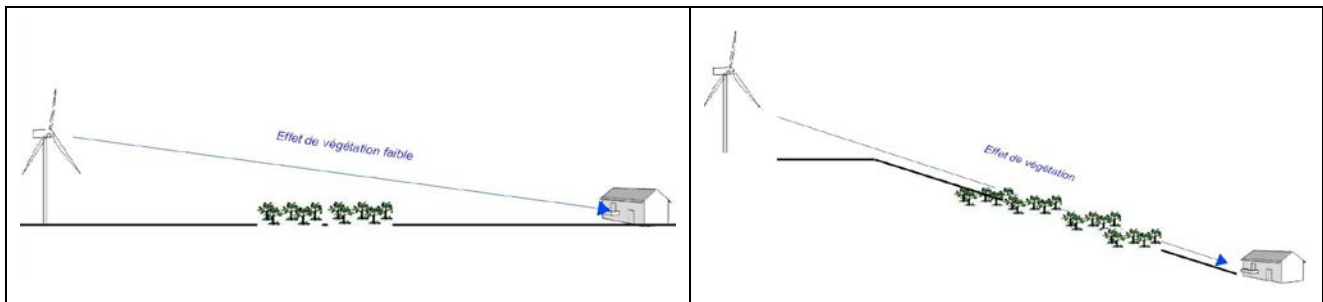
Figure 45 : influence de l'effet de végétation lorsque la source apparente est haute (à gauche : effet négligeable) et basse (à droite : effet possible)
