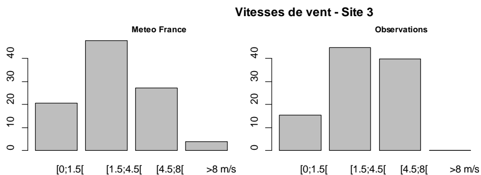
Figure 114 : roses des vents à 10 m de hauteur
