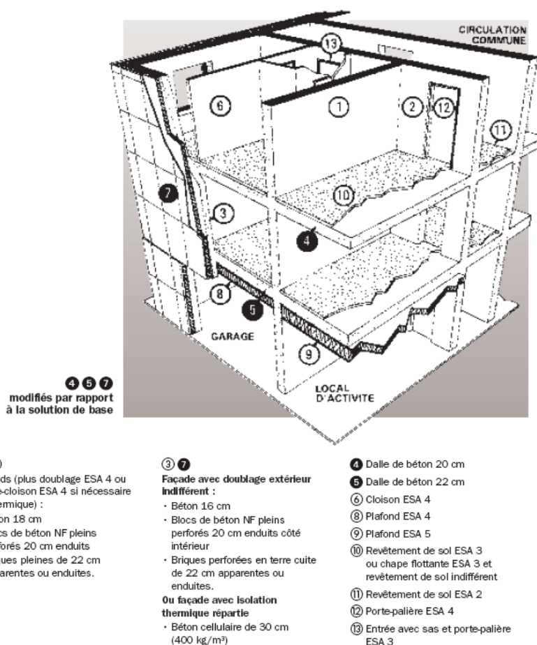
Figure 4.2.4 Extrait des Exemples de Solutions Acoustiques (DGUHC - 2002)
