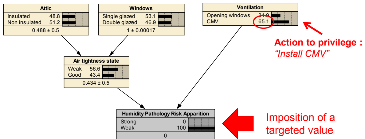
Figure 8 - Exemple d'imposition d'une valeur-cible sur un indicateur, et propagation de l'information jusqu'aux procédés techniques à mettre en œuvre (structure bayésienne simplifiée pour l'exemple)
