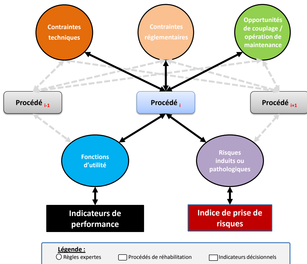
Figure 6 - Architecture et dépendances des différents types de règles expertes avec les procédés de réhabilitation et les indicateurs de performance globale
