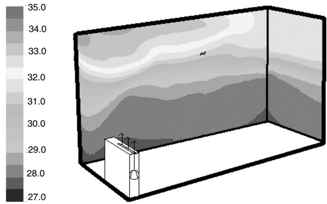
Figure 5 : Simulation détaillée du profil de température à 5 cm des murs Ventilo-convecteur, chauffage, basse vitesse de ventilation
